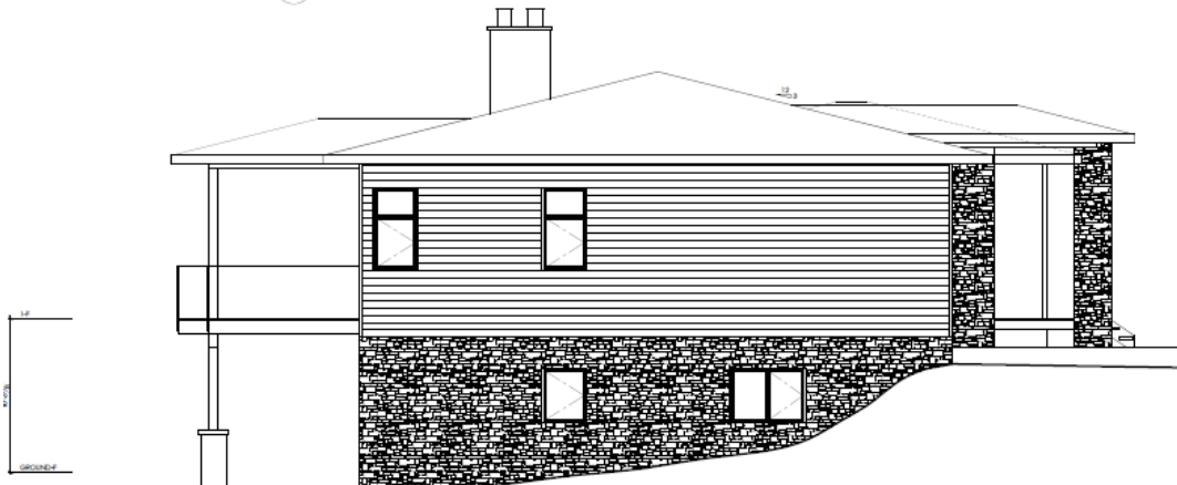
2 SIDE ELEVATION A-5
